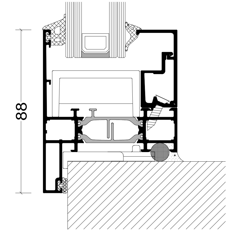
AANSLUITING ONDER
