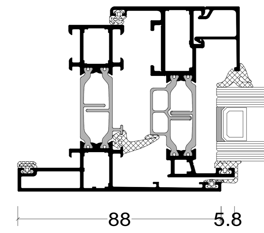
STANDAARD VLEUGEL
