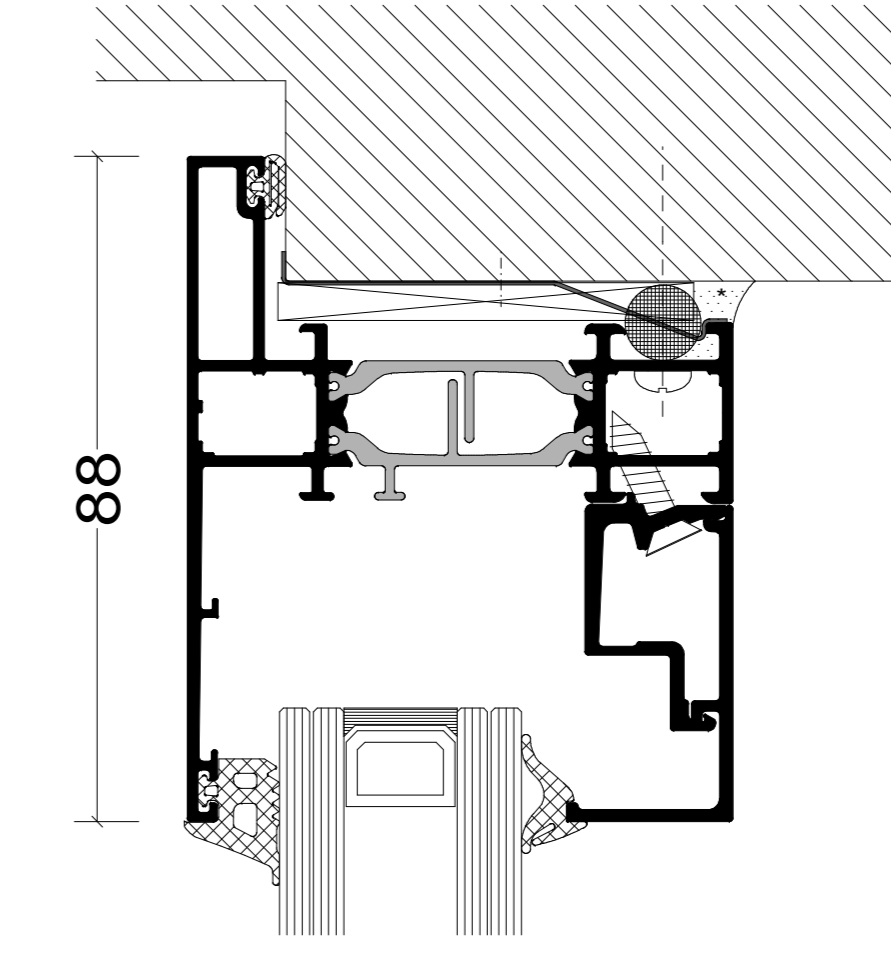
AANSLUITING BOVEN
