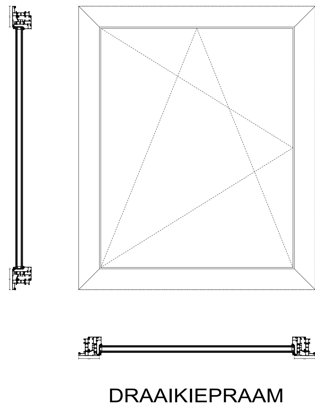
DRAAIKIEPRAAM
