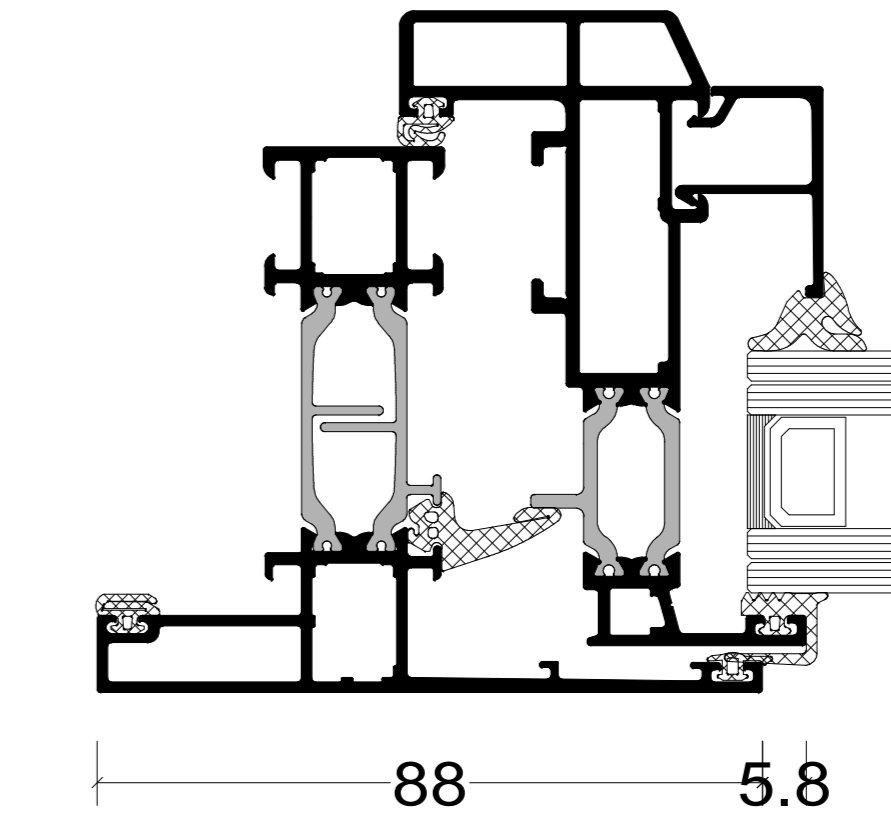
SOFTLINE VLEUGEL
