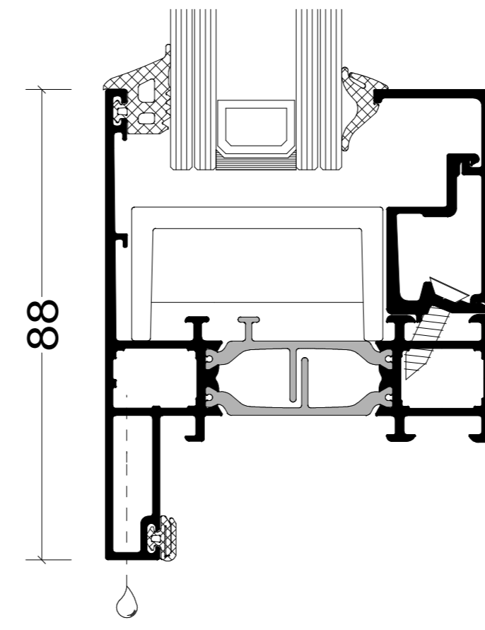
VERBORGEN WATERAFVOER
