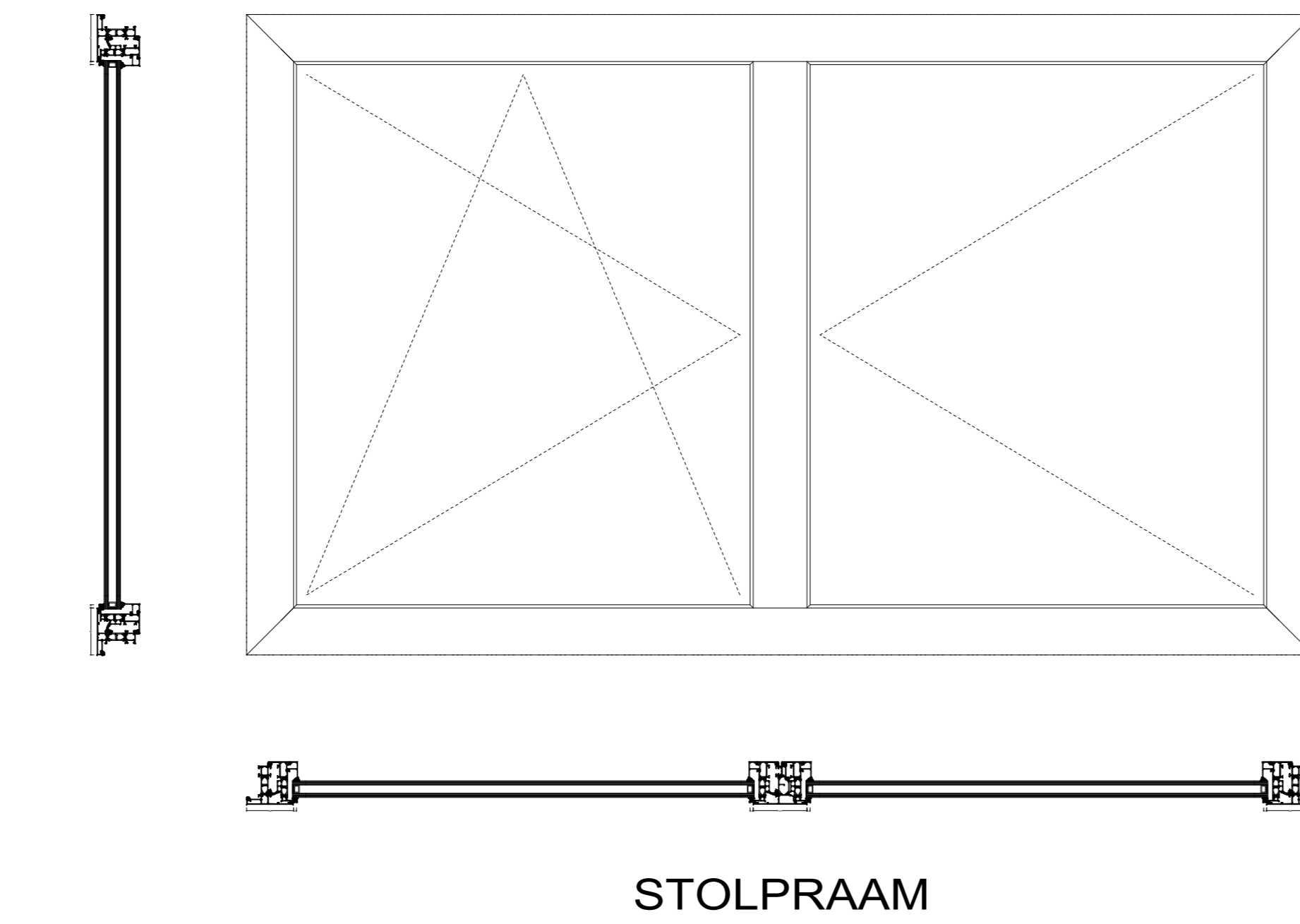
STOLPRAAM
