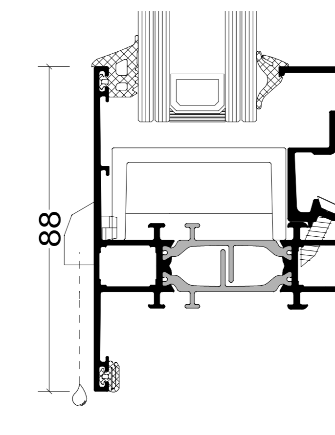
GECOMPARTIMENTEERDE WATERAFVOER
