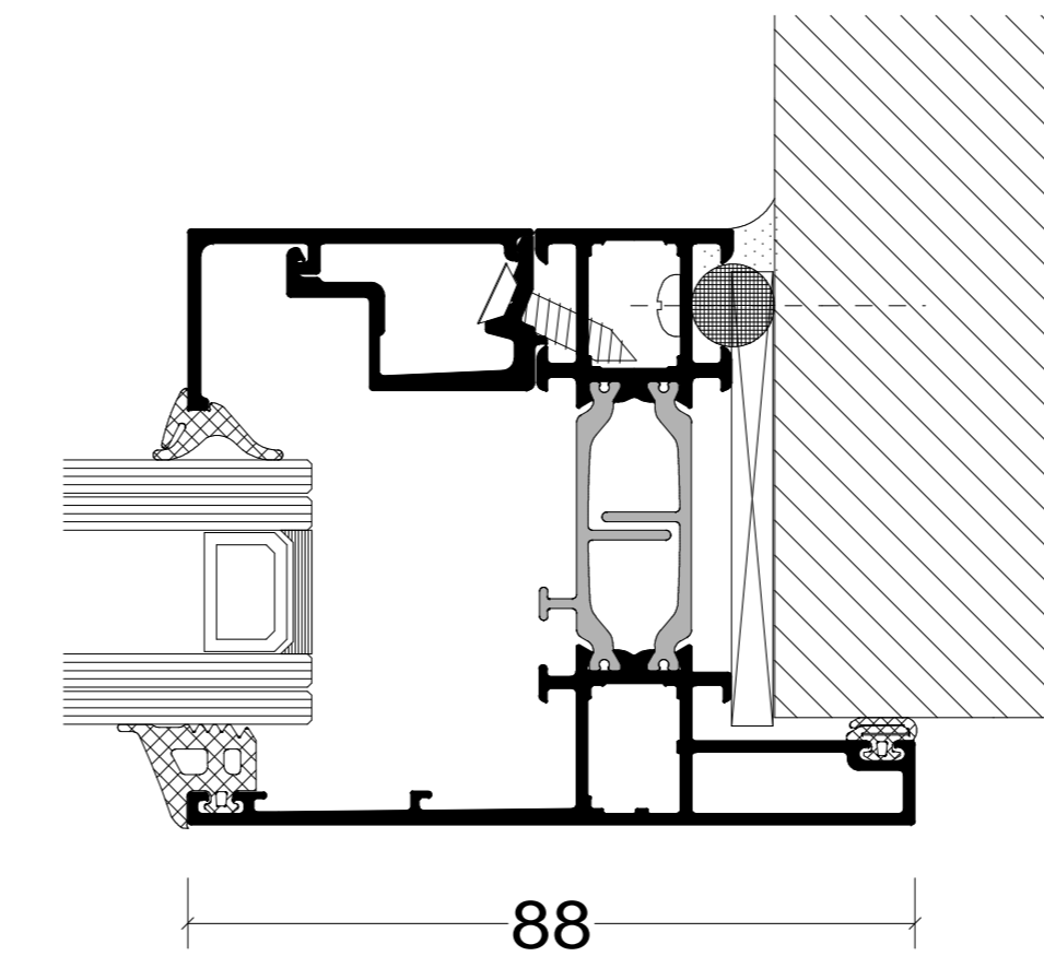
AANSLUITING ZIJ
